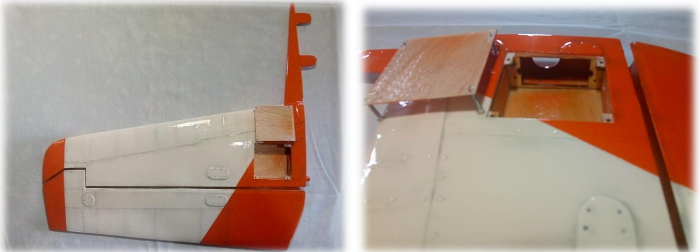
Acima: Localização da tampa de acesso ao servo do profundor(esquerda) e base de fixação do servo (direita).
